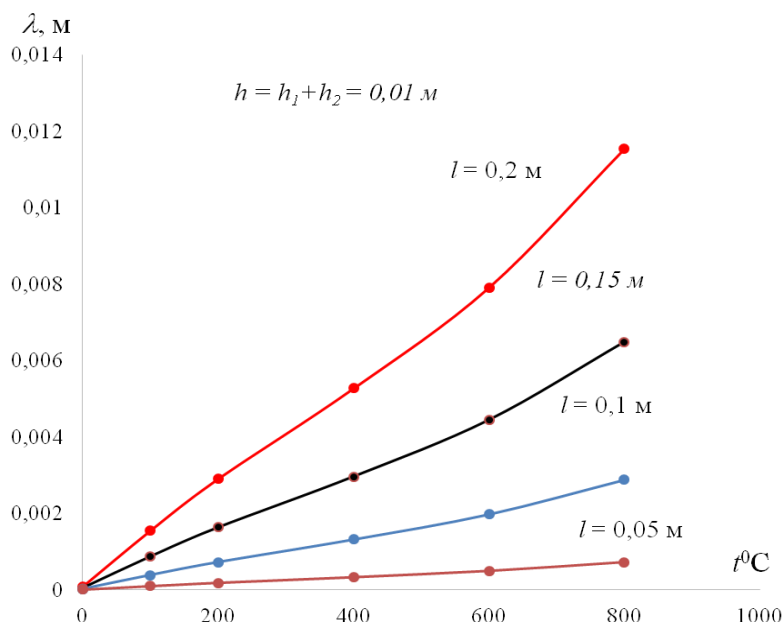
Рис. 3. Влияние температуры и длины на прогиб при нагреве биметалла на \Delta t = 5 ^{\circ}\text{C}
