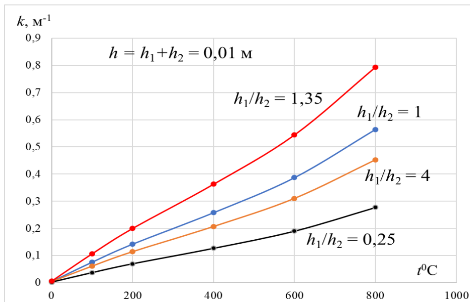
Рис. 2. Влияние температуры и толщины слоев на кривизну при нагреве биметалла на \Delta t = 5 °С
