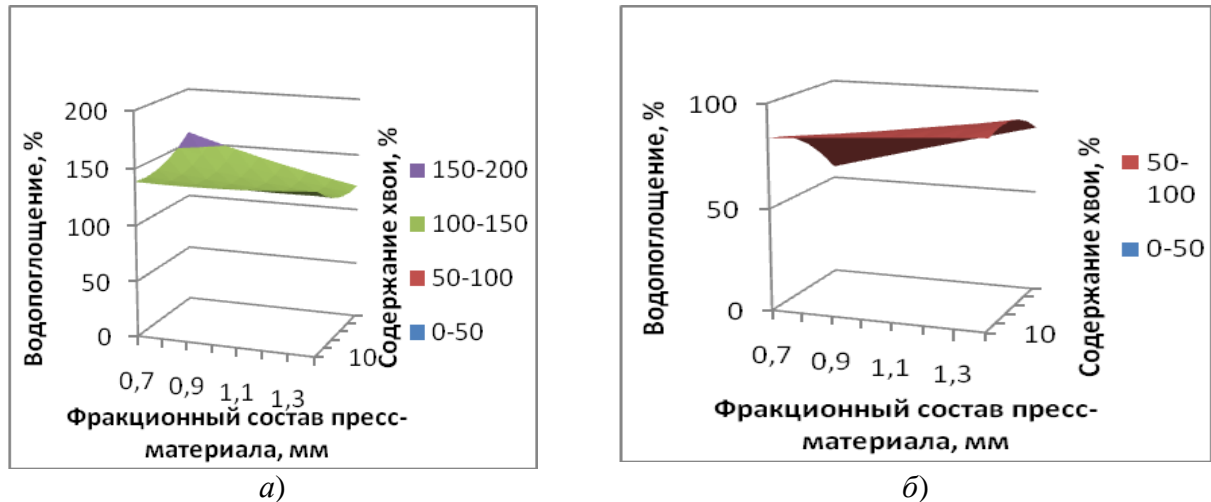
Рис. 2. Поверхность зависимости водопоглощения ДП-БС от содержания в хвое и фракционного состава пресс-сырья: а — ДП-БС сухая хвоя сосны; б — ДП-БС сухая хвоя лиственницы
