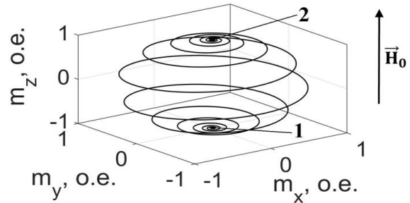
Рис. 2. Фазовый портрет движения вектора намагниченности
